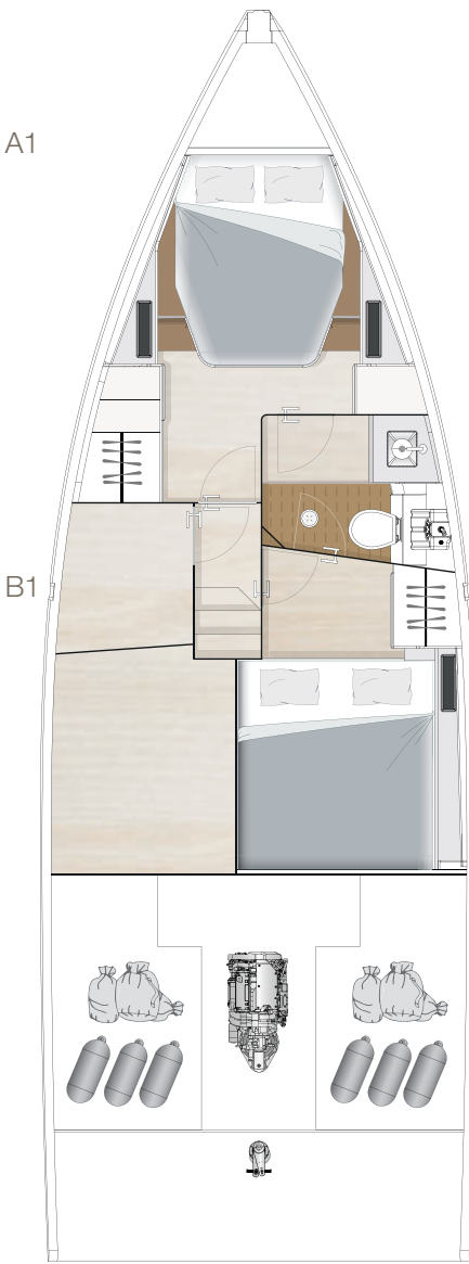
Lowerdeck standard
