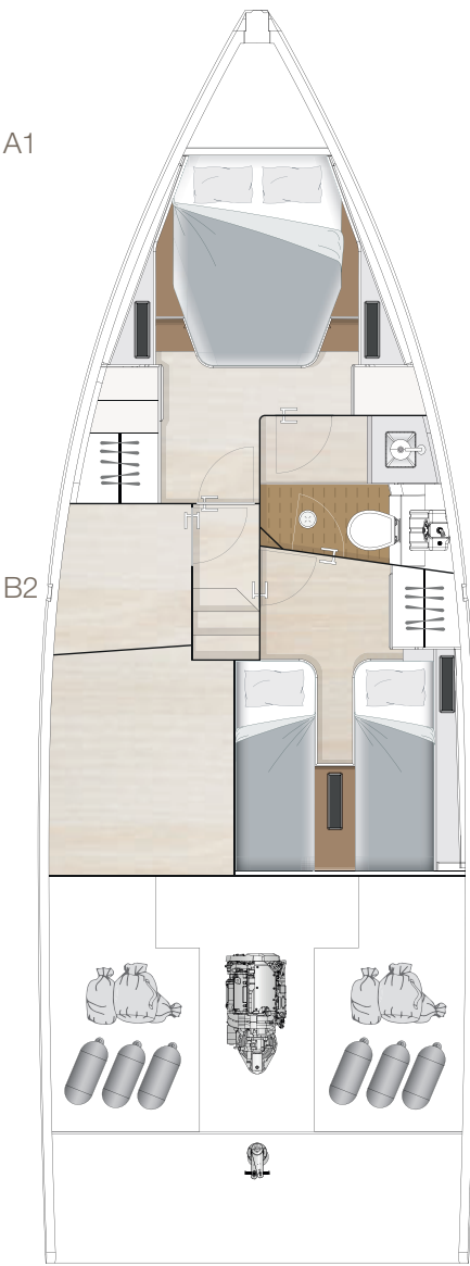
Lowerdeck option
